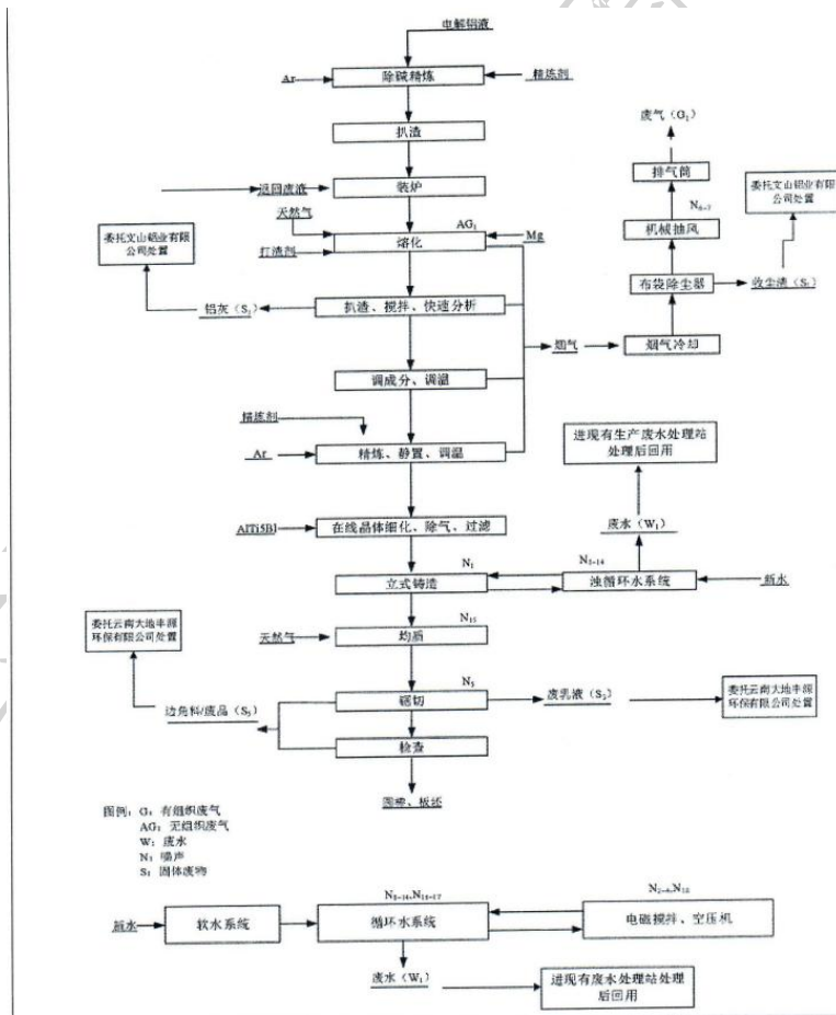
图 2 排放单位工艺流程图
