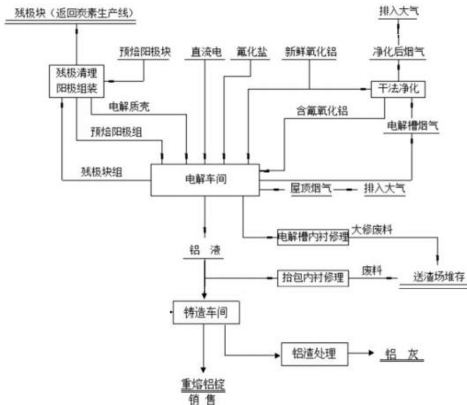
图 2 排放单位电解工艺流程图
